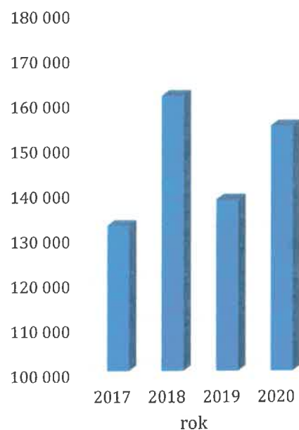
Vlastní kapitál
