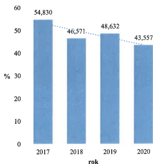
Celková zadluženost
