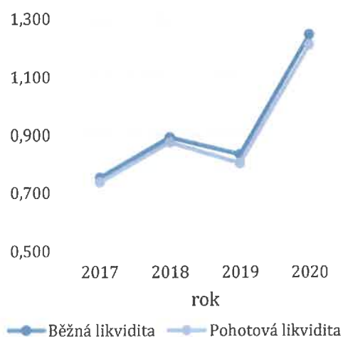
Vývoj likvidity
